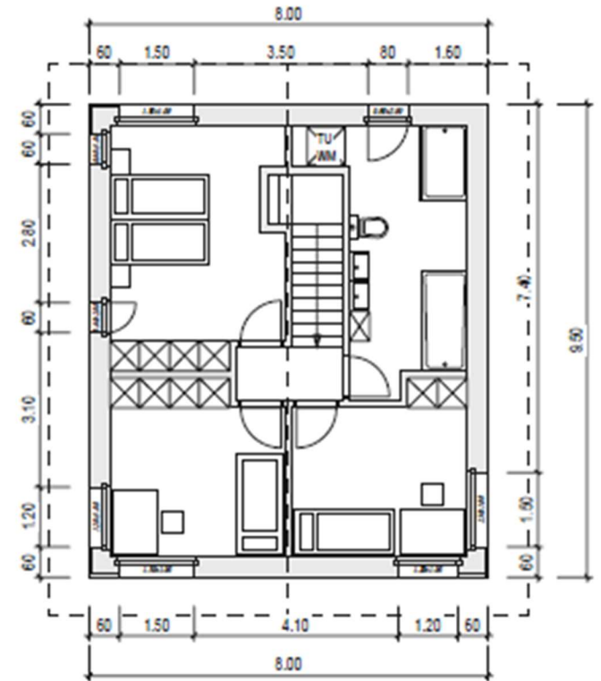
Grundriss OG
