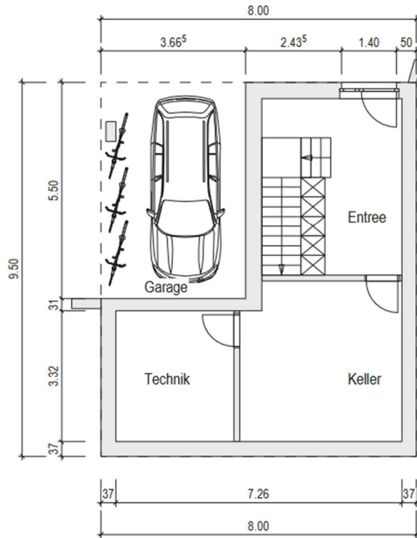
Grundriss UG
