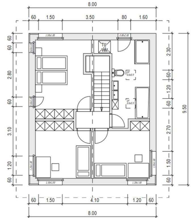
Grundriss OG
