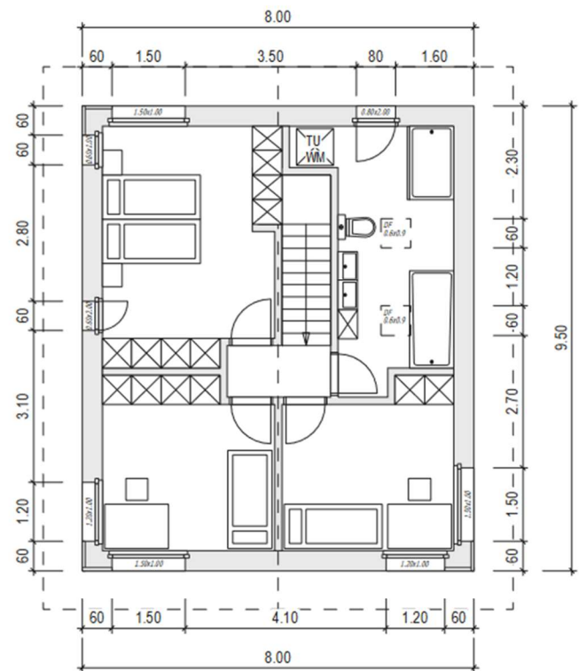
Grundriss OG
