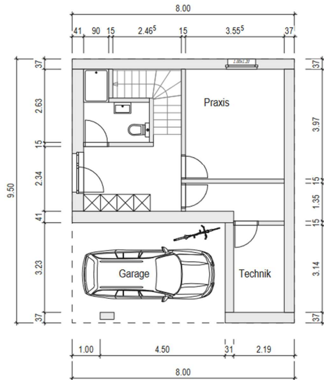
Grundriss UG
