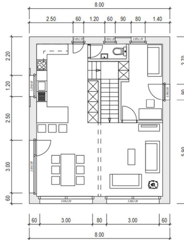
Grundriss EG
