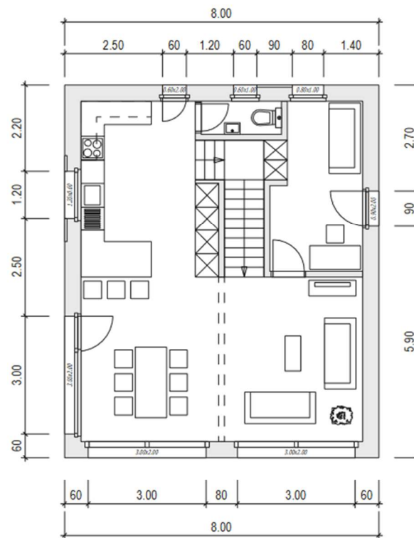
Grundriss EG
