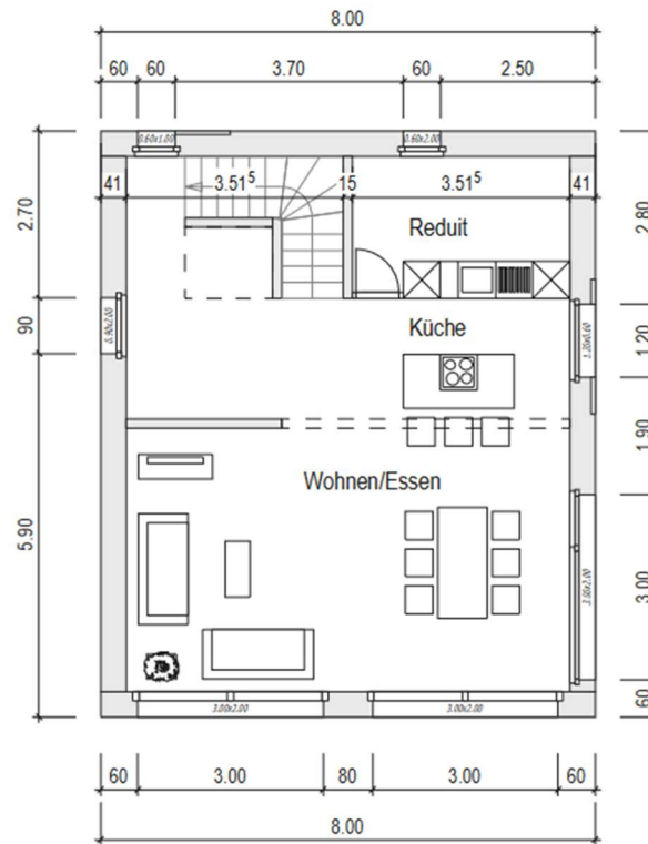
Grundriss EG
